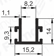
Pr.No: 3492 0,154 kg/m
