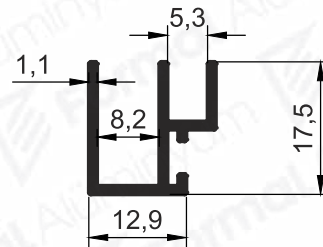
Pr.No: 3493 0,189 kg/m
