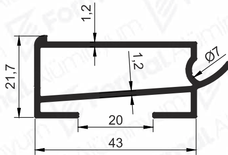
Pr.No: 4411 0,509 kg/m
