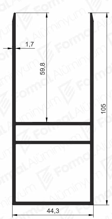
Pr.No: 2612 1,477 kg/m
