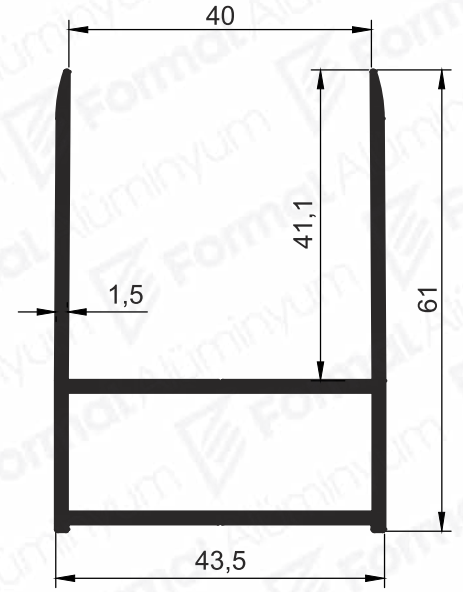
Pr.No: 2692 0,813 kg/m
