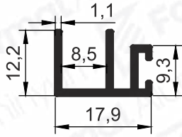
Pr.No: 2956 0,159 kg/m
