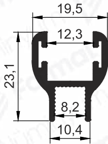
Pr.No: 2406 0,263 kg/m
