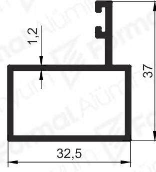
Pr.No: 1921 0,420 kg/m
