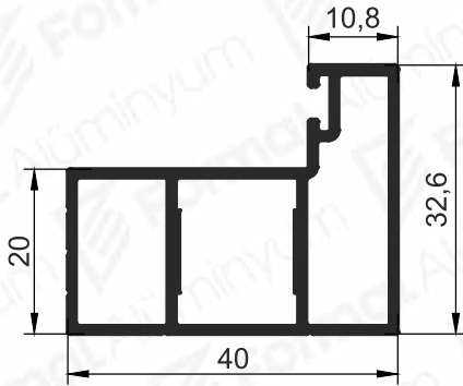
Pr.No: 4081 0,518 kg/m
