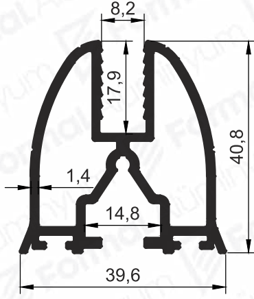
Pr.No: 5158 0,833 kg/m
