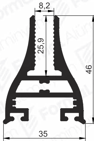
Pr.No: 9620 1,009 kg/m
