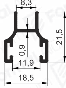
Pr.No: 5261 0,173 kg/m
