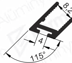
Pr.No: 3513 0,132 kg/m
