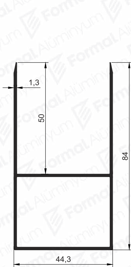
Pr.No: 5362 0,854 kg/m
