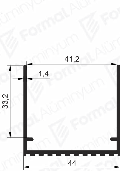
Pr.No: 2336 0,532 kg/m
