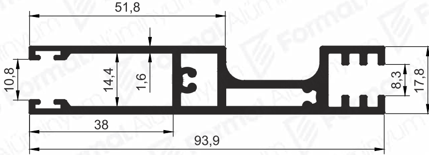
Pr.No: 2955 1,288 kg/m
