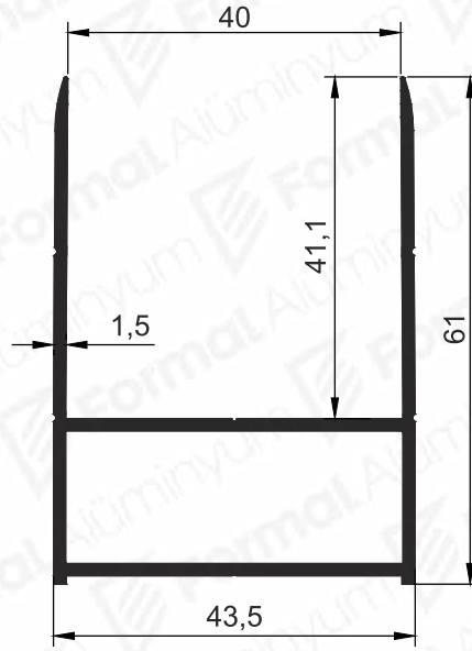
Pr.No: 1817 0,811 kg/m
