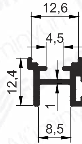
Pr.No: 2957 0,141 kg/m
