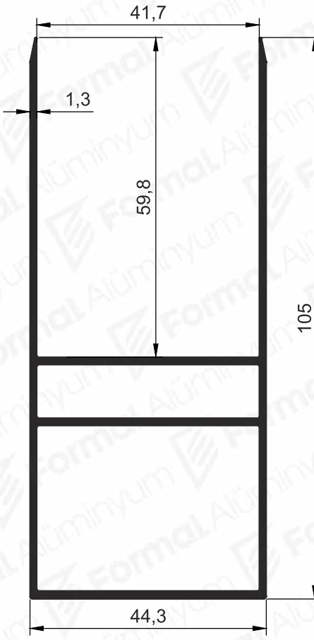
Pr.No: 3848 1,214 kg/m
